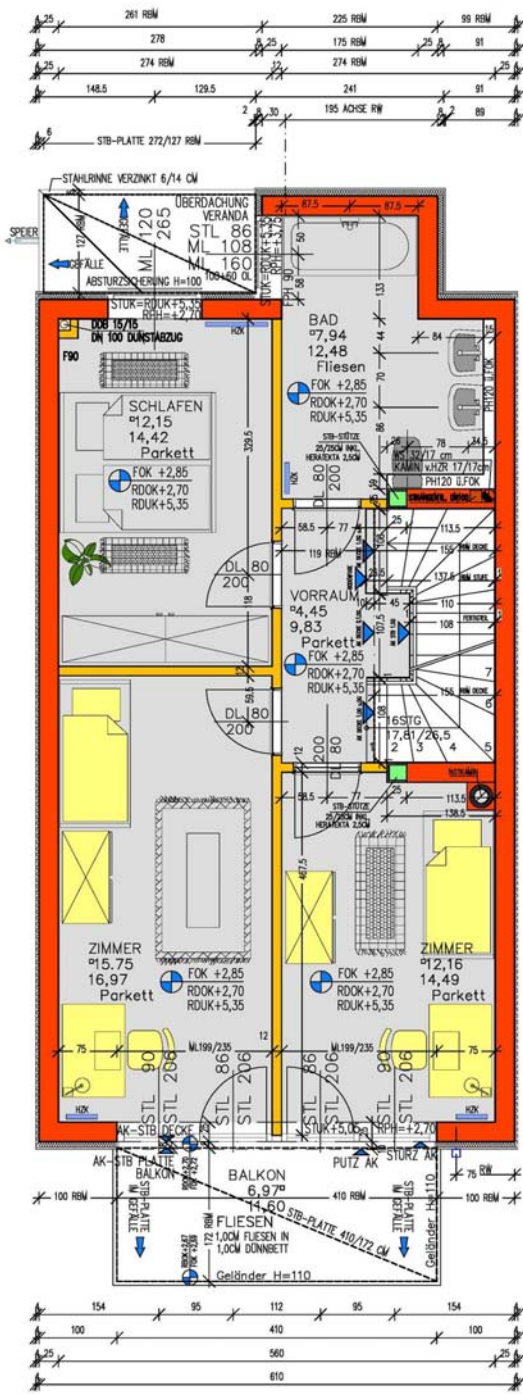
Grundriss OG Bauteil A/B
